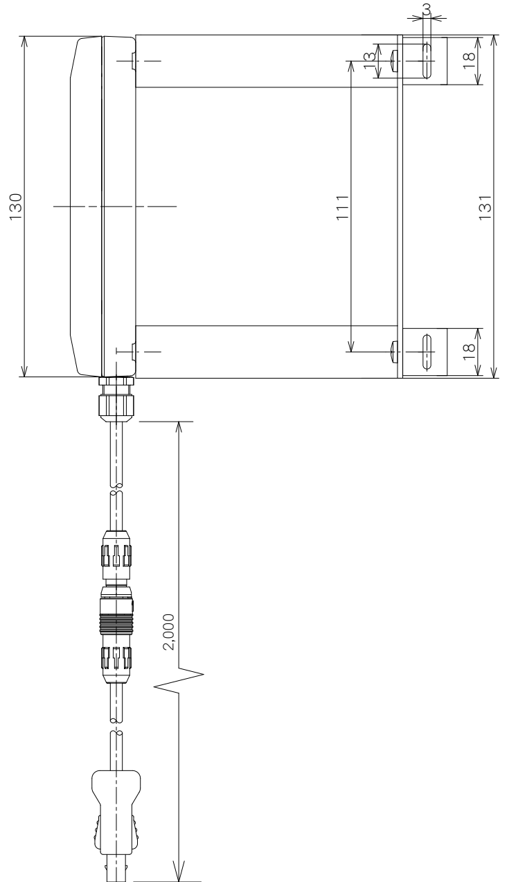
UMM-□□□□ホ-ル取付金具組込み寸法図
