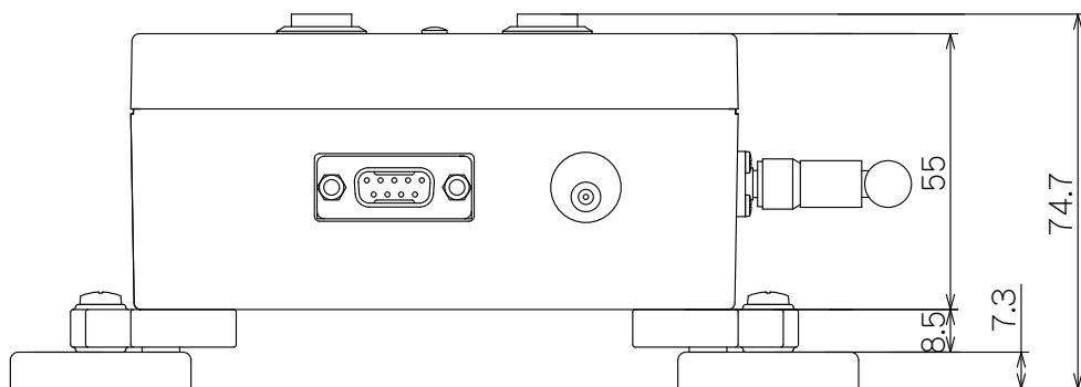
FCall-M8S マグネット付 外観寸法図
