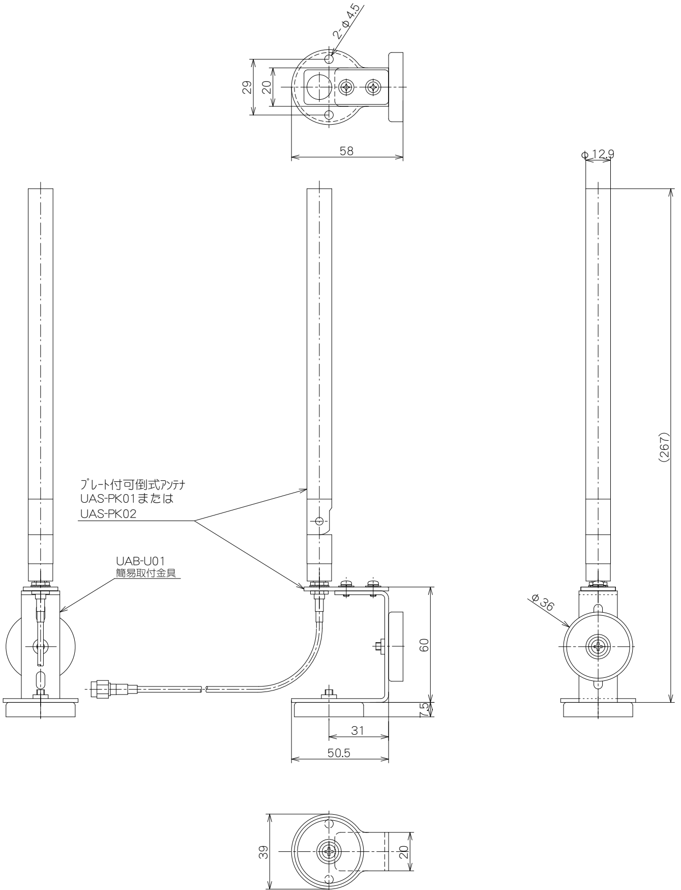
プレート付可倒式アンテナ & 簡易取付金具外觀寸法図
