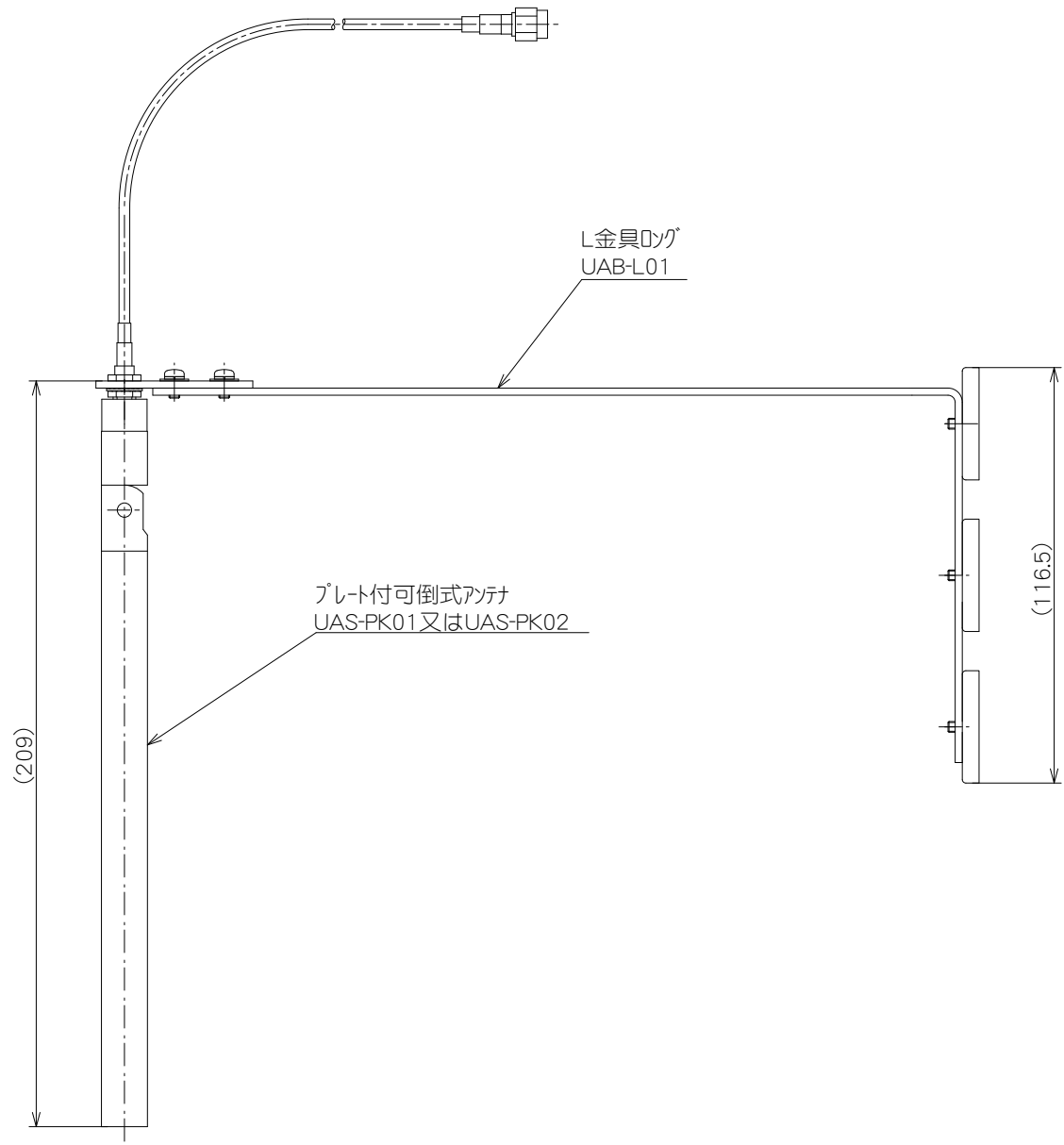
【アンテナ下向き取付】
