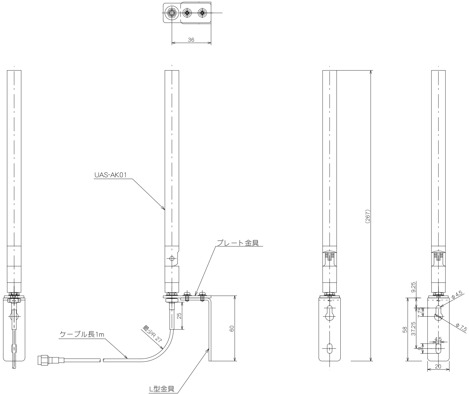
UAS-PK01 プレート付アンテナ外觀寸法図 Rev1.0
